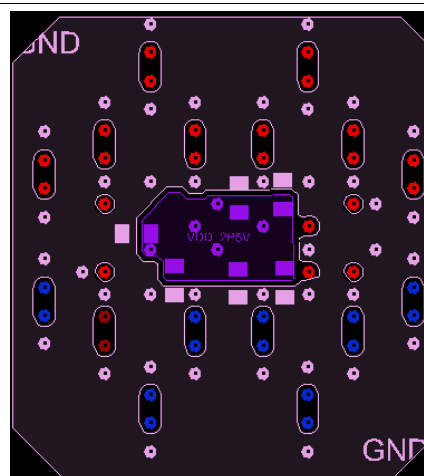
Figure 23. Bottom Layer
