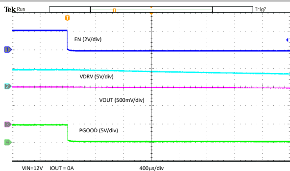
Figure 7-11. EN Shutdown
