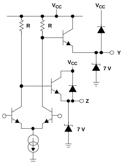
OUTPUT LVP20
