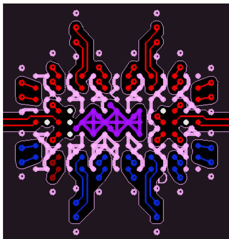
Figure 29. Top Layer
