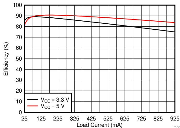
SN6505A-Q1 + Würth 750315240
