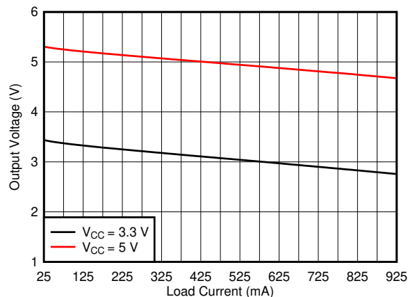
SN6505A-Q1 + Würth 750315240
