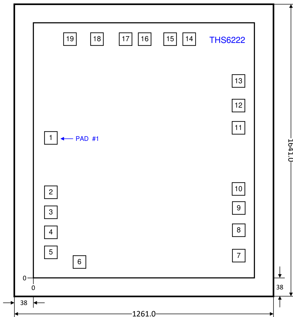
Figure 7-4. Die Dimensions
