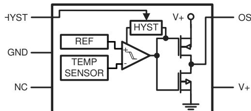
Figure 6-2. LM26CIM5 - __ E
