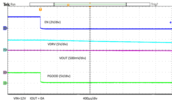
Figure 7-11. EN Shutdown
