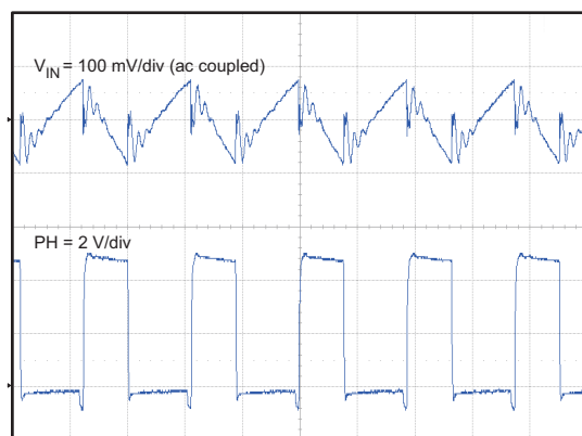
INPUT RIPPLE, 5 A
