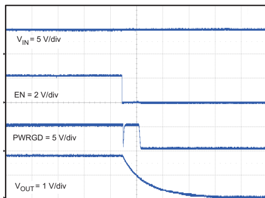
POWER DOWN VOUT, EN
