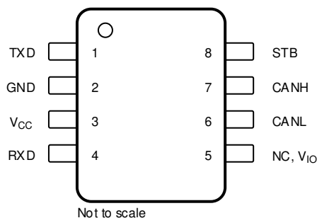
Figure 4-1. SOIC (D) and SOT-23 (DDF) Package, 8 Pin (Top View)
