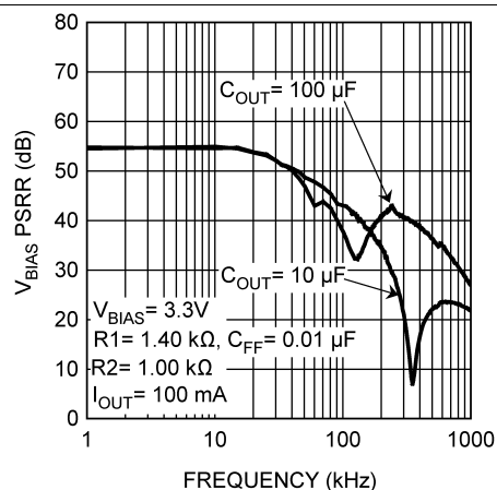
Figure 19. V_{BIAS} PSRR
