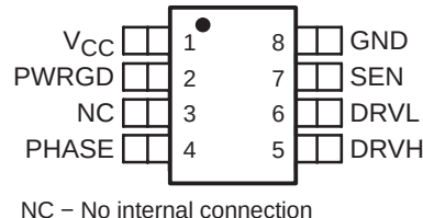
SO (D) PACKAGE (TOP VIEW)
