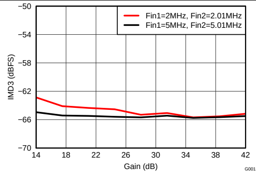
Figure 45. IMD3
