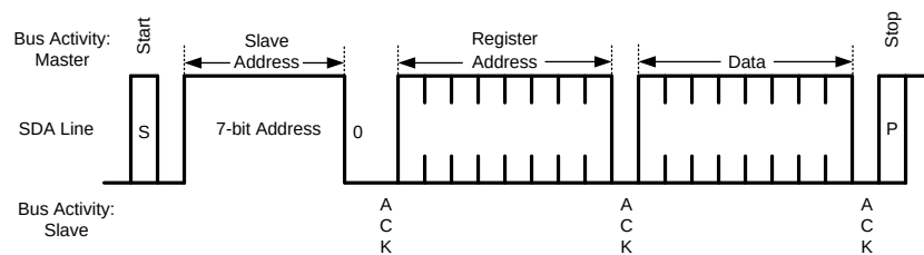
Figure 24. Write Byte
