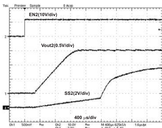
Figure 11. VO2=1.5V, SoftStart
