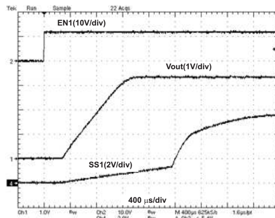
Figure 10. VO1=3.3V, SoftStart
