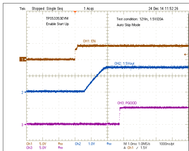
Figure 8-2. Enable Turnon
