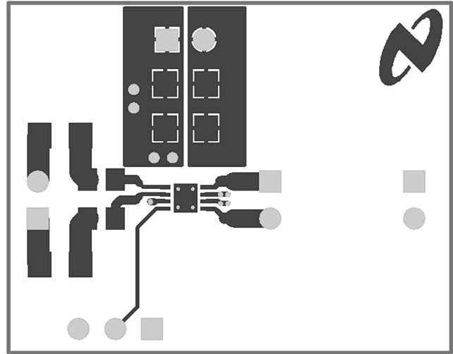
Internal Layer 1
