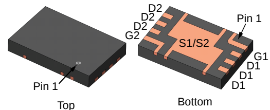
PQFN8 3.3X5, 0.65P (Power 3.3 x 5) CASE 483AU
