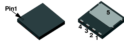
PQFN 8x8, 2P (Power88) CASE 483AP
