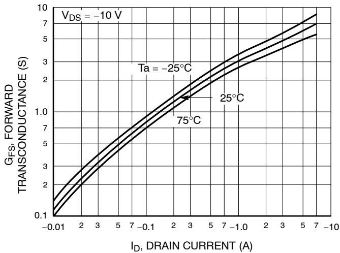
Figure 6. g_{FS} - I_D
