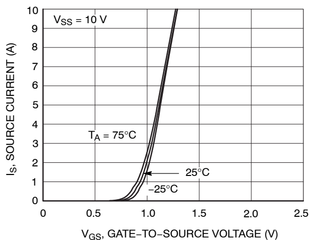
Figure 9. I_S - V_{GS}
