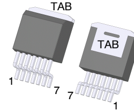
TO-263-7 CASE 418BA
