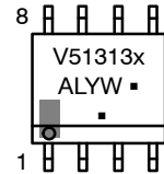
SOIC-8 NB CASE 751-07
