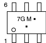
SOT-363 CASE 419B
