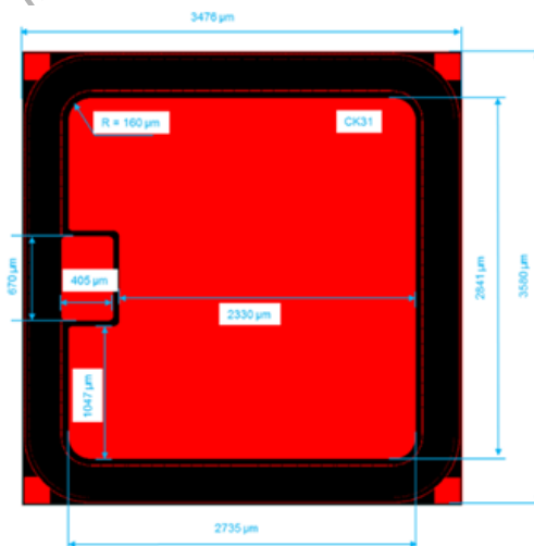
DIE OUTLINE
