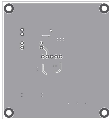
Figure 3—Bottom Layer
