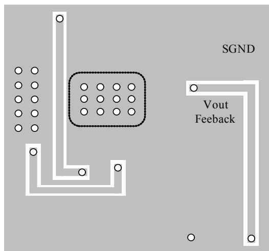
Bottom Layer
