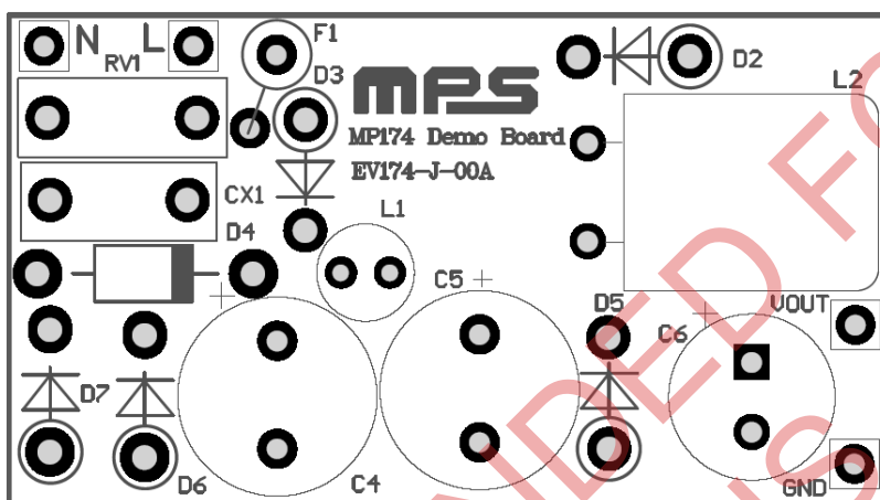
Figure 2—Top Layer
