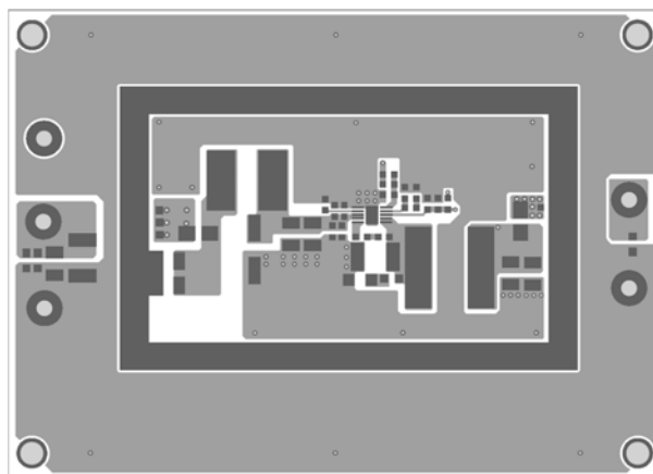
Figure 2—Top Layer
