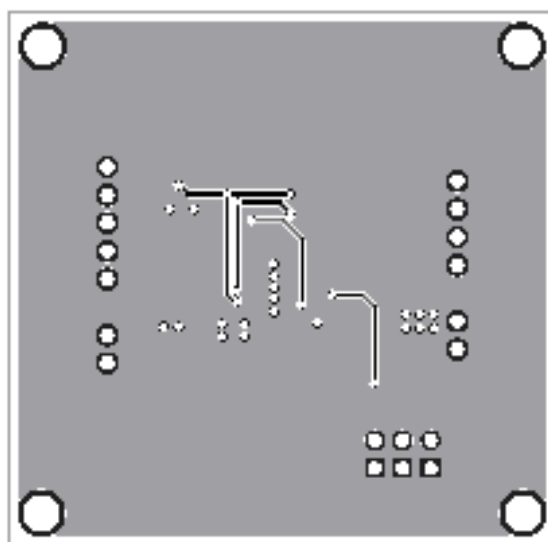
Figure 3—Bottom Layer
