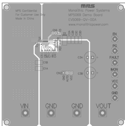
Figure 1—Top Layer
