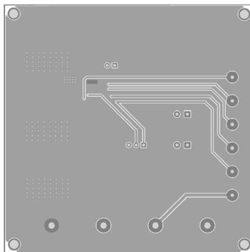
Figure 2—Bottom Layer
