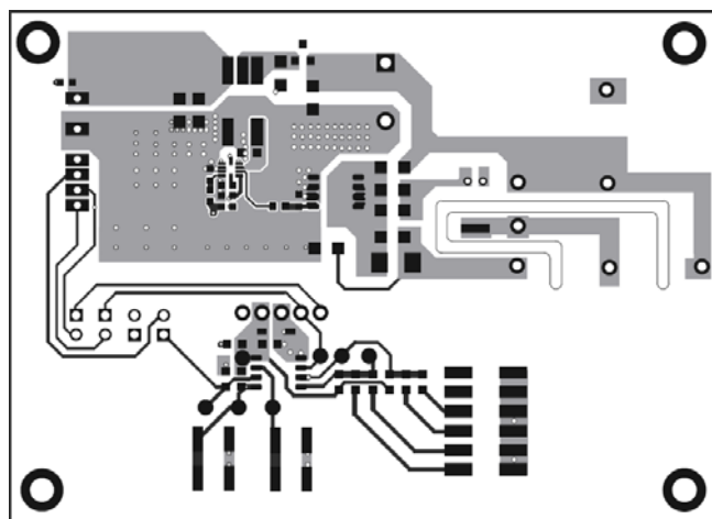
Figure 2—Top Layer
