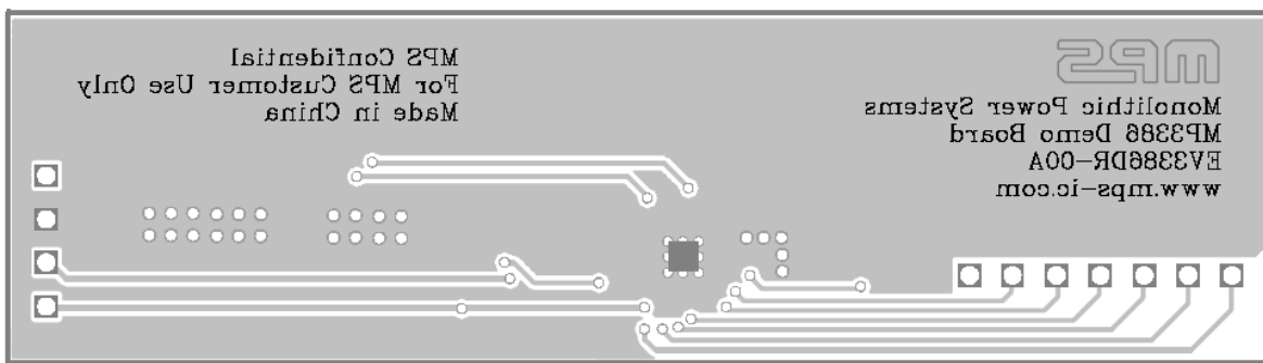
Figure 2—Bottom Layer
