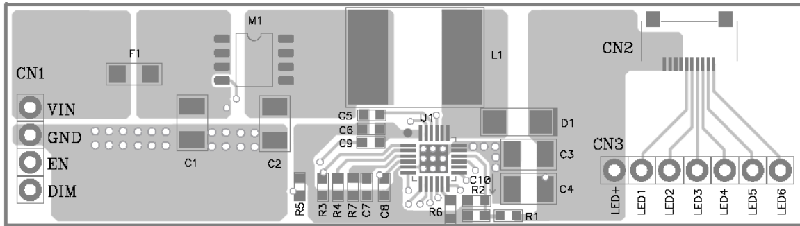
Figure 1—Top Layer
