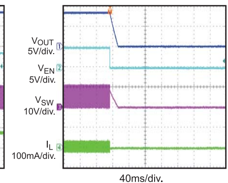
EN Shutdown
