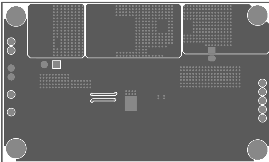
Figure 2—Bottom Layer
