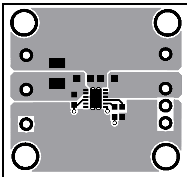
Figure 2—Top Layer
