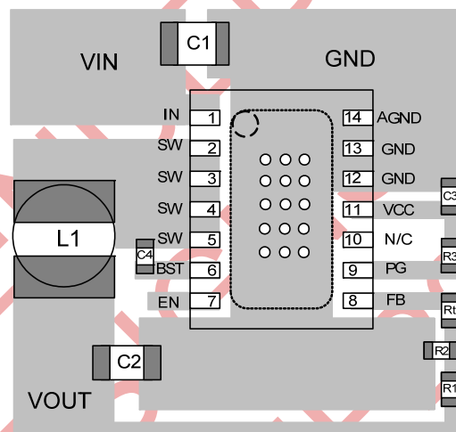
Top Layer
