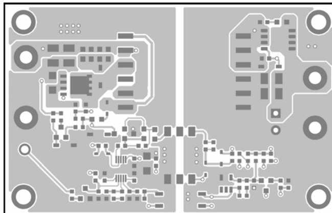
Figure 2—Top Layer
