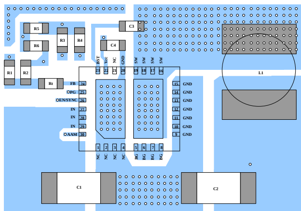
Top Layer
