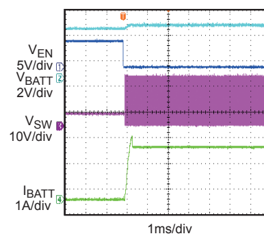
EN On Waveform
