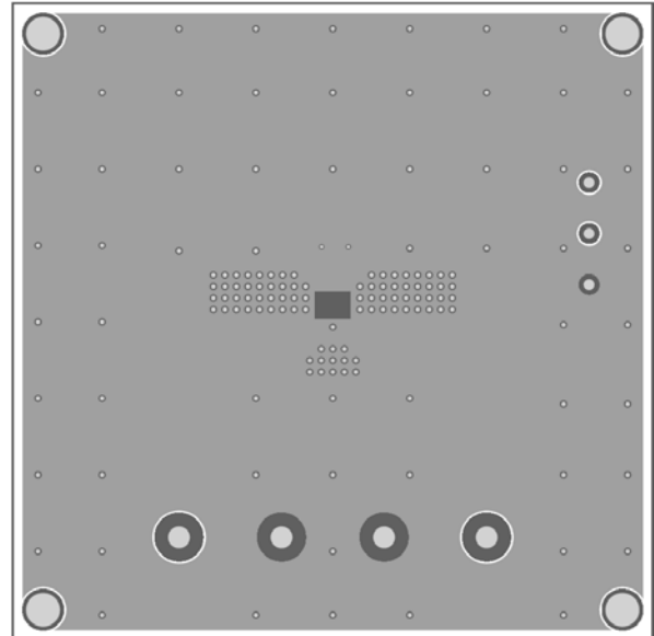
Figure 2—Bottom Layer
