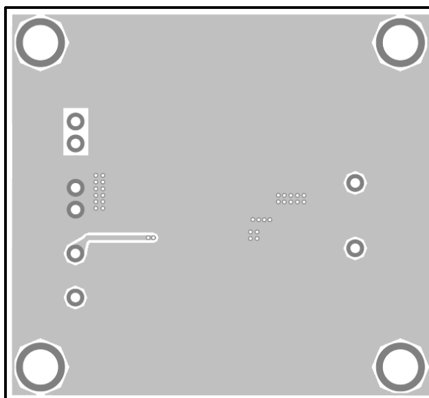
Figure 2—Bottom Layer
