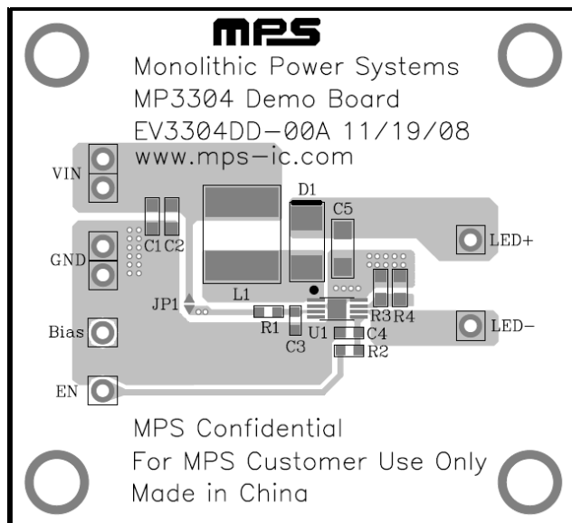
Figure 1—Top Layer
