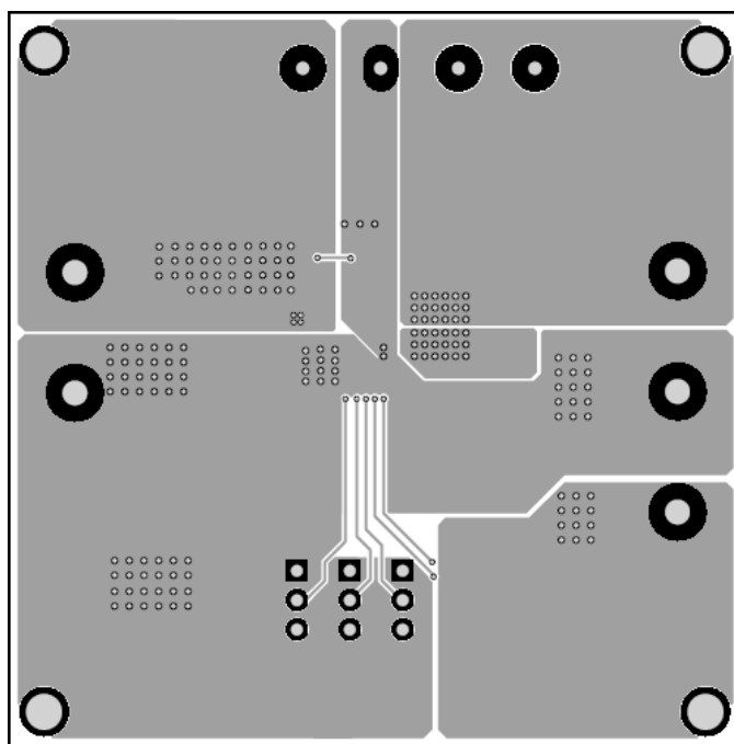
Figure 3—Bottom Layer
