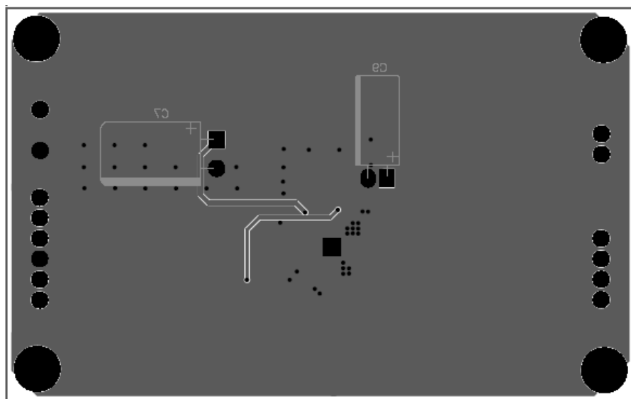
Figure 2—Bottom Layer
