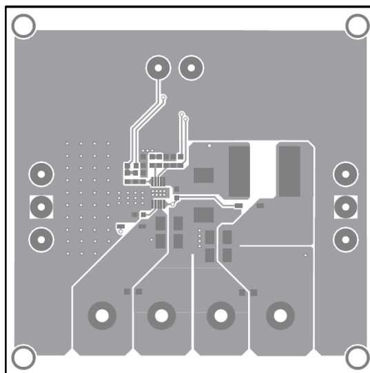
Figure 2—Top Layer
