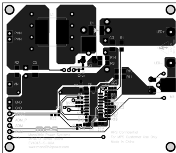
Figure 2—Top Layer
