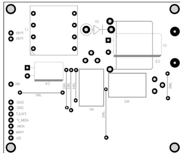
Figure 4—Bottom Layer
