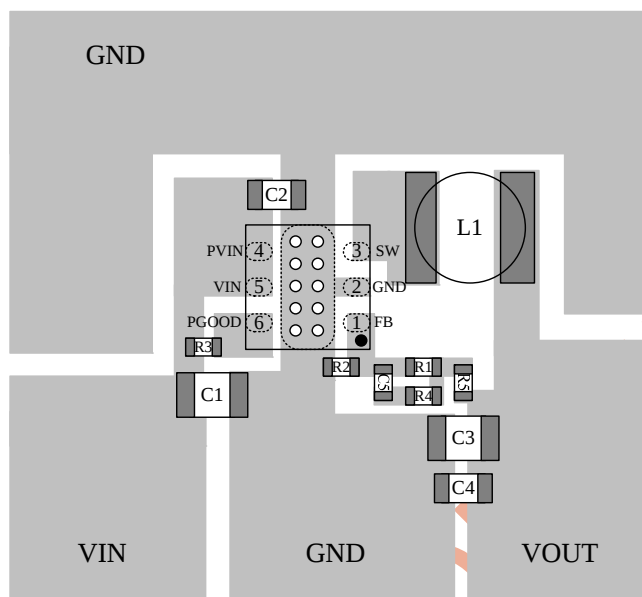
Top Layer
