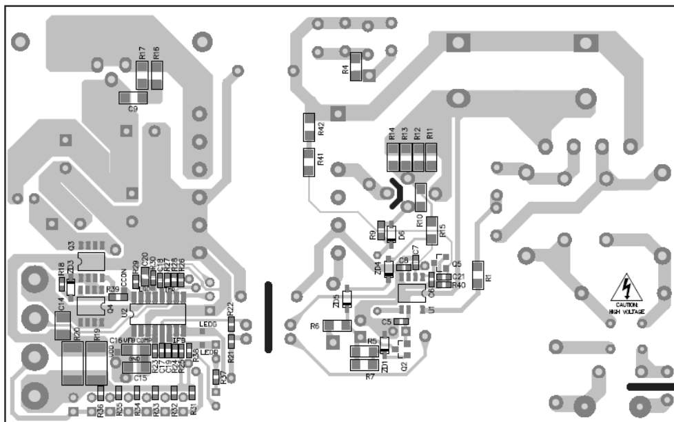
Figure 2—Bottom Layer
