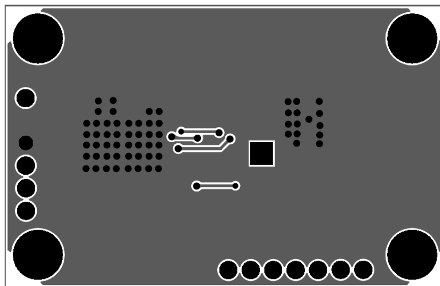
Figure 2—Bottom Layer
