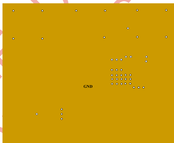
Inner1 Layer
